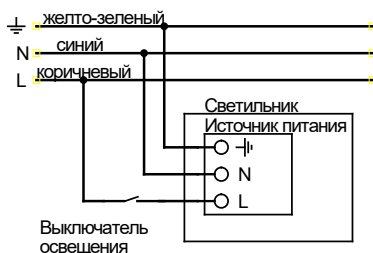
Рис.1. Схема подключения
