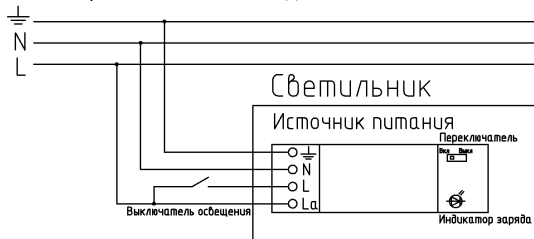
Рис.1. Схема подключения
