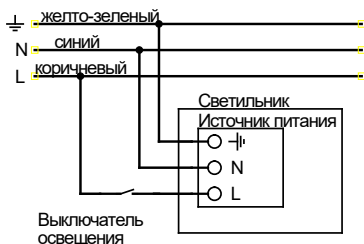
Рис.1. Схема подключения
